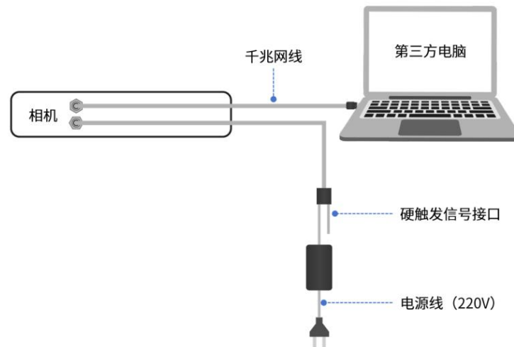
图 2-1 Mark 相机线缆连接示意图
