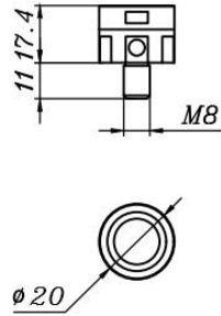
图 1-3 Mark 灯 20mm 尺寸图
