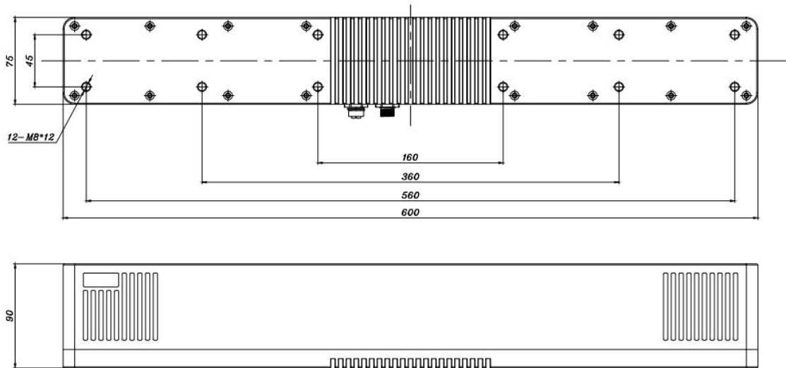
图 1-1 520 瞳距 Mark 相机尺寸示意图
