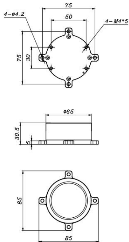
图 1-4 Mark 灯 50mm 尺寸图
