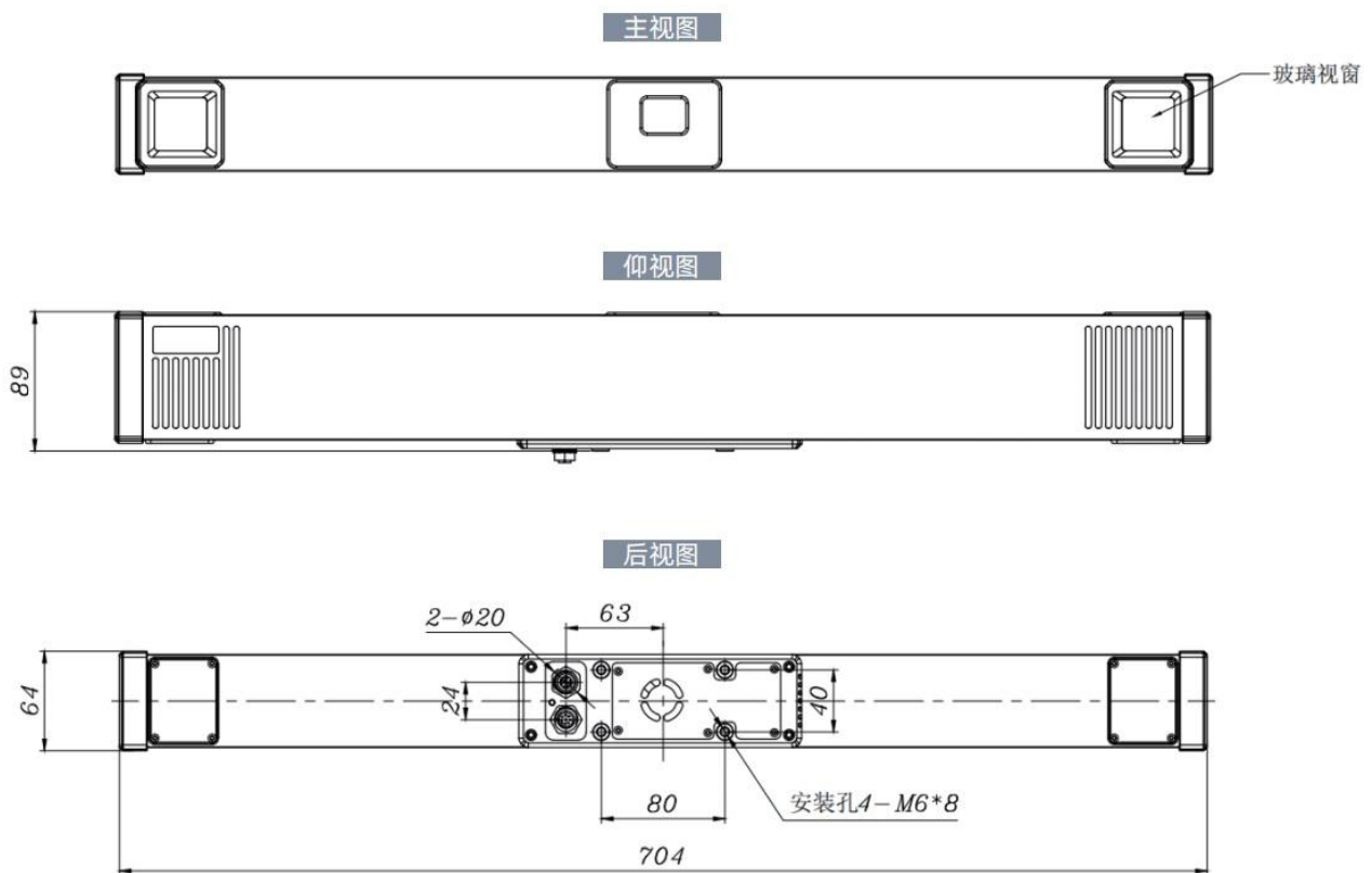
图 1-2 620 瞳距 Mark 相机尺寸示意图
