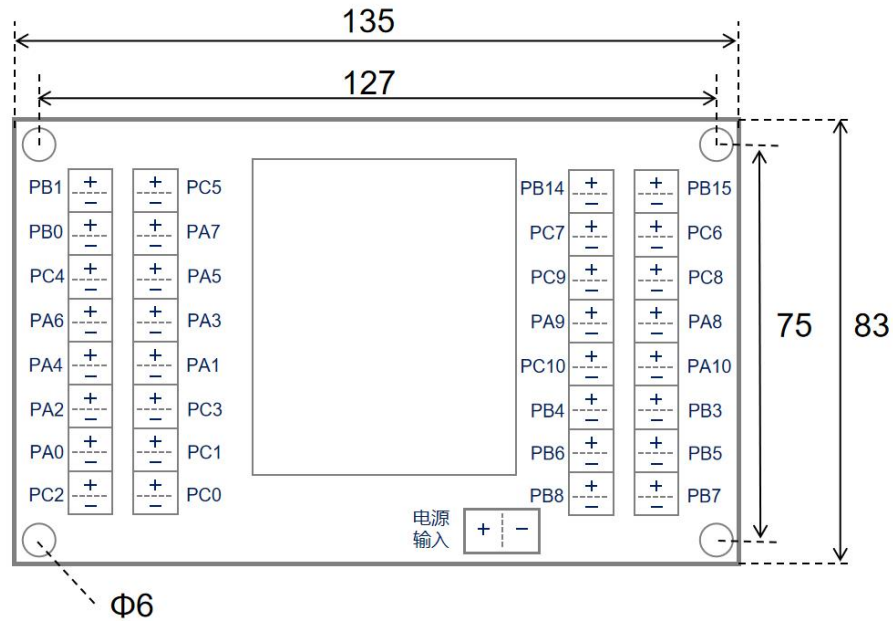
图 1-5 Mark 灯控制板尺寸图
