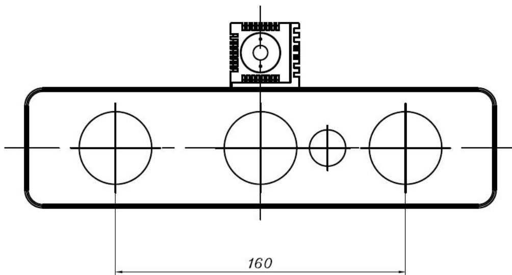
正视图
