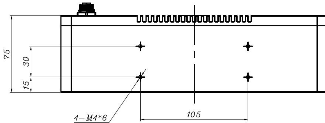
俯视图
