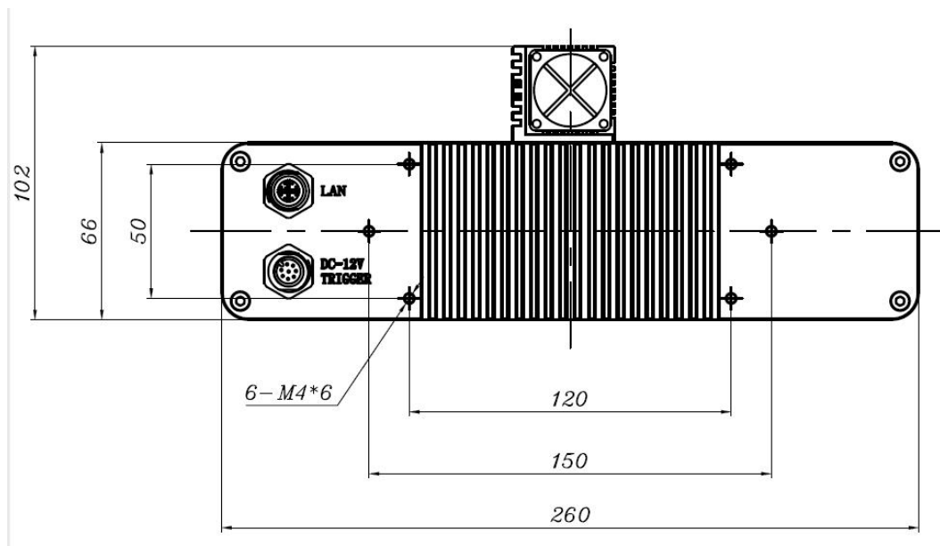
后视图
